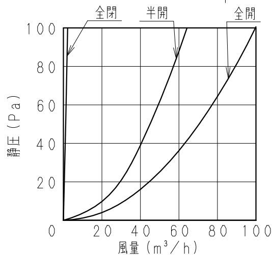
■抵抗損失曲線
