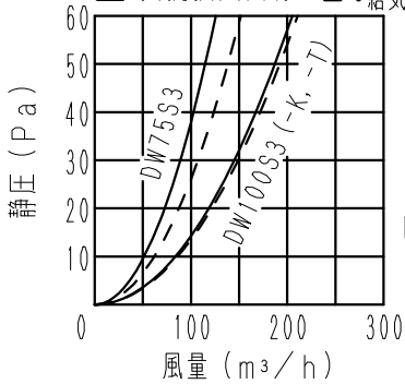
■ 抵抗損失曲線
