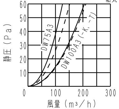
■抵抗損失曲線
