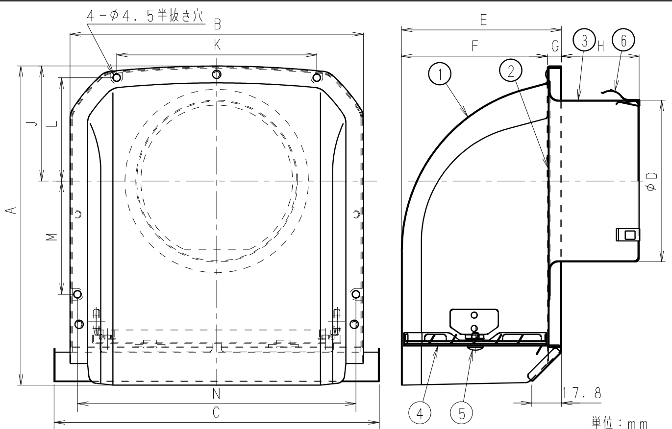
■寸法表
