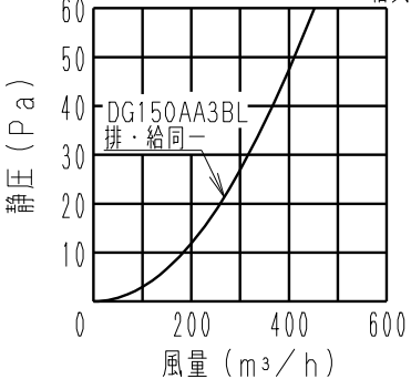
■抵抗損失曲線 ー 排気 ー 給気
