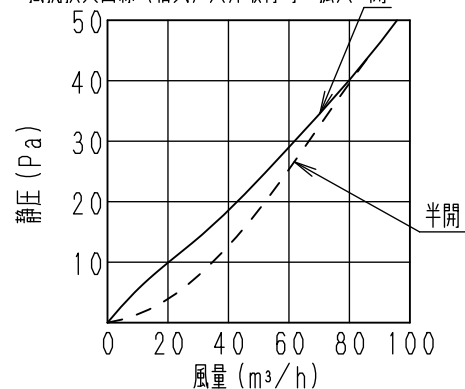
■抵抗損失曲線（給気）天井取付時 拡大
