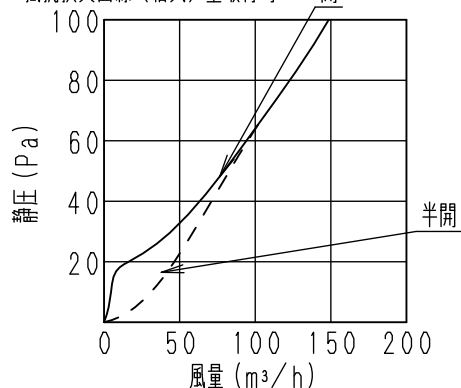
■抵抗損失曲線（給気）壁取付時 拡大
