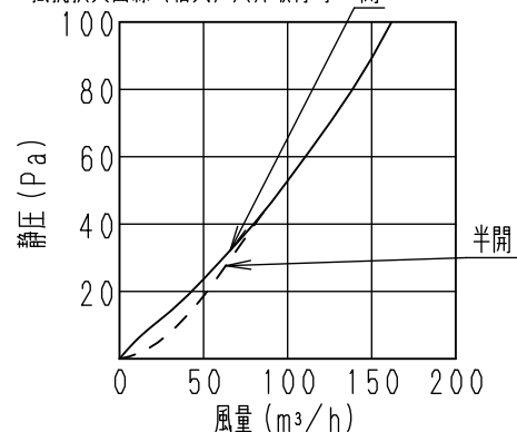
■抵抗損失曲線（給気）天井取付時 拡大
