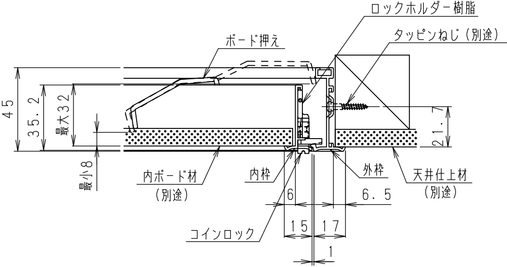
木製天井下地断面納まり図（１：２）
